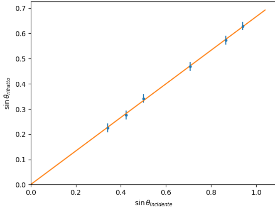
Figura 2: Interpolazione lineare passante per l'origine tra \sin \theta_{\text{inc}} e \sin \theta_{\text{rif}} .
